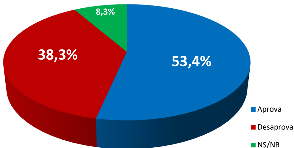
Gráfico 2 – Aprovação da Gestão do Prefeito Rodrigo Drable
