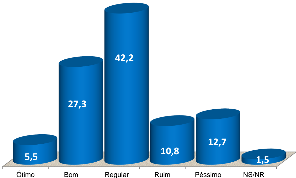
Gráfico 1 - Avaliação do Rodrigo Drable (%)
