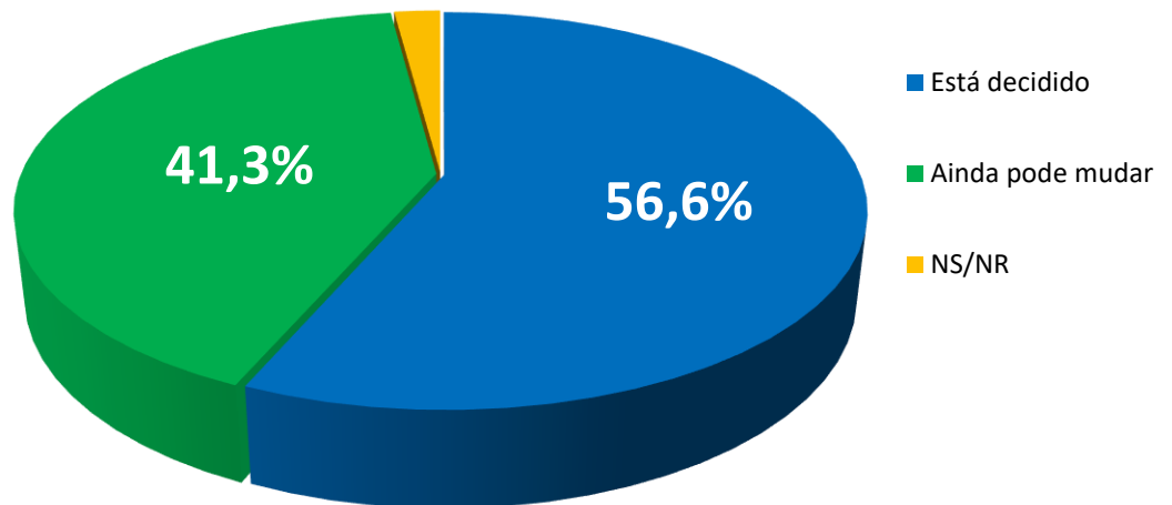
Gráfico 6 - Decisão sobre o Voto: Está decidido X Ainda pode mudar
