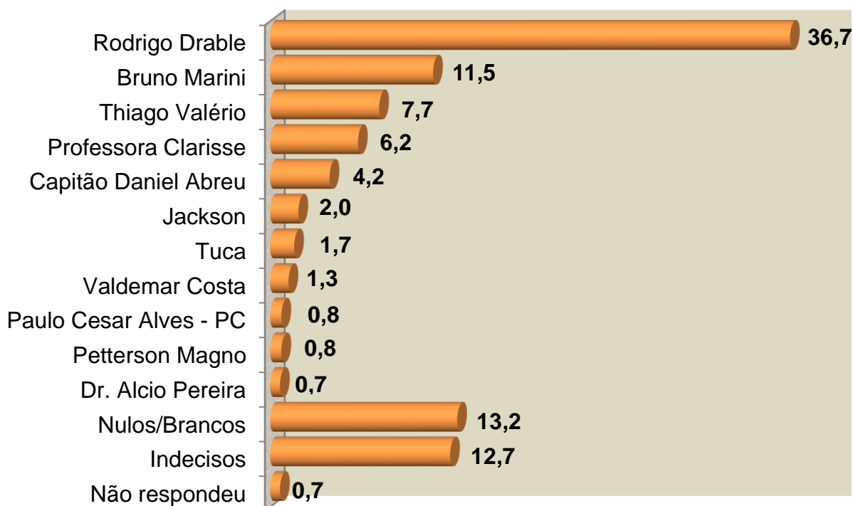
Gráfico 5 – Intenção de Voto para PREFEITO DE BARRA MANSA - Estimulada (%)
