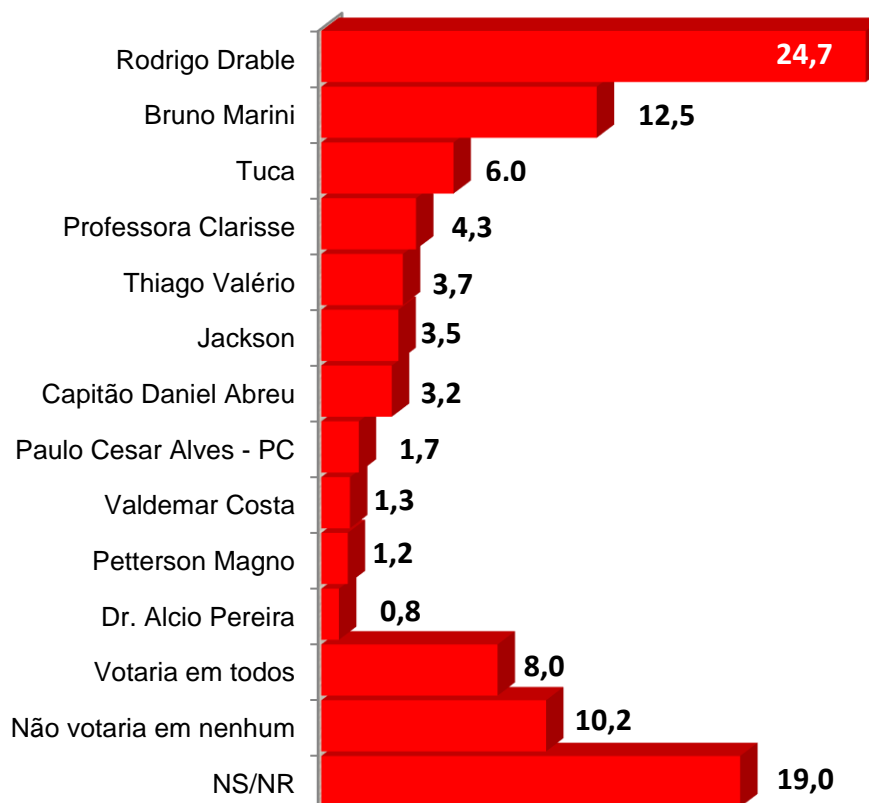
Gráfico 7 - Rejeição para PREFEITO (%)
