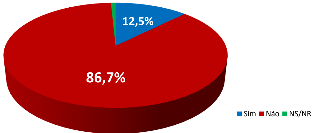
Gráfico 4 – Simpatia por algum partido político? (%)
